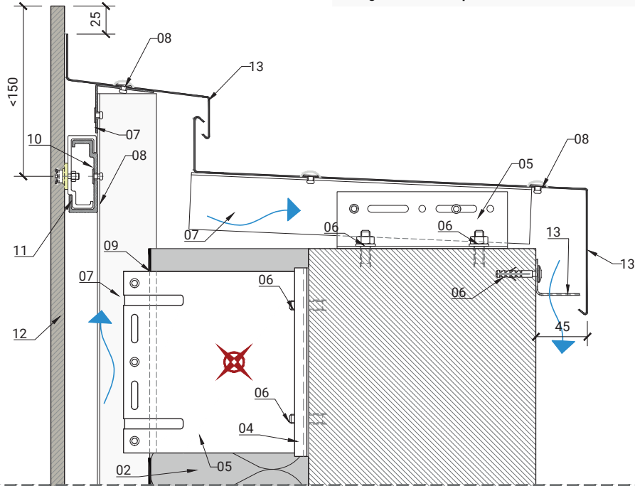
Dettaglio H2-16 Parapetto con lattoneria
