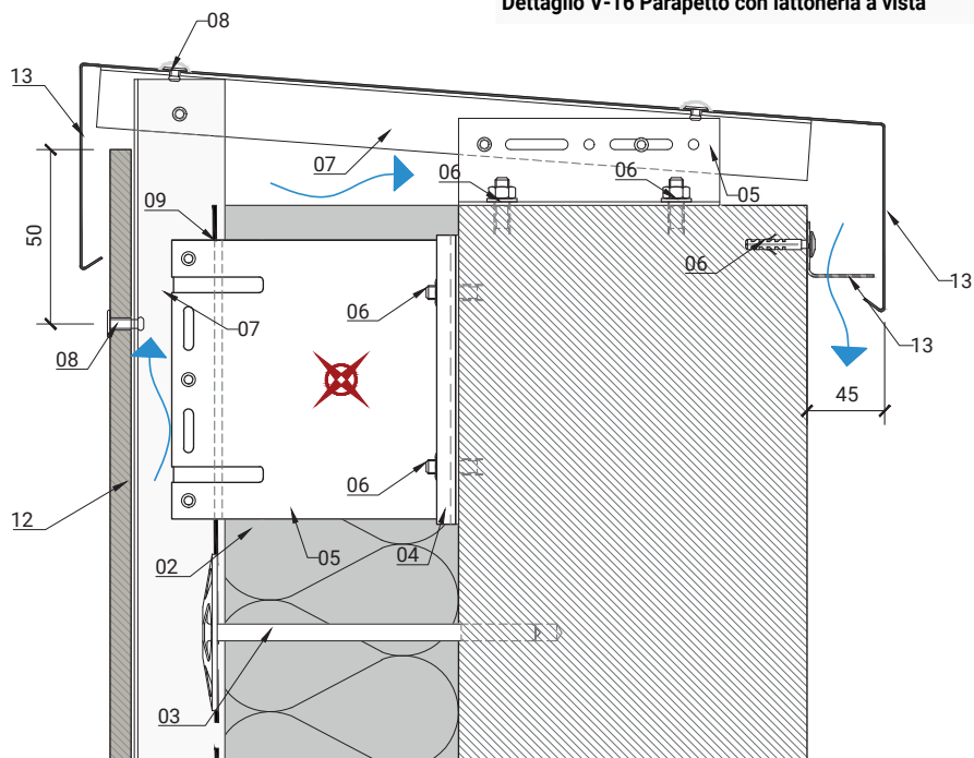
Dettaglio V-16 Parapetto con latteneria a vista
