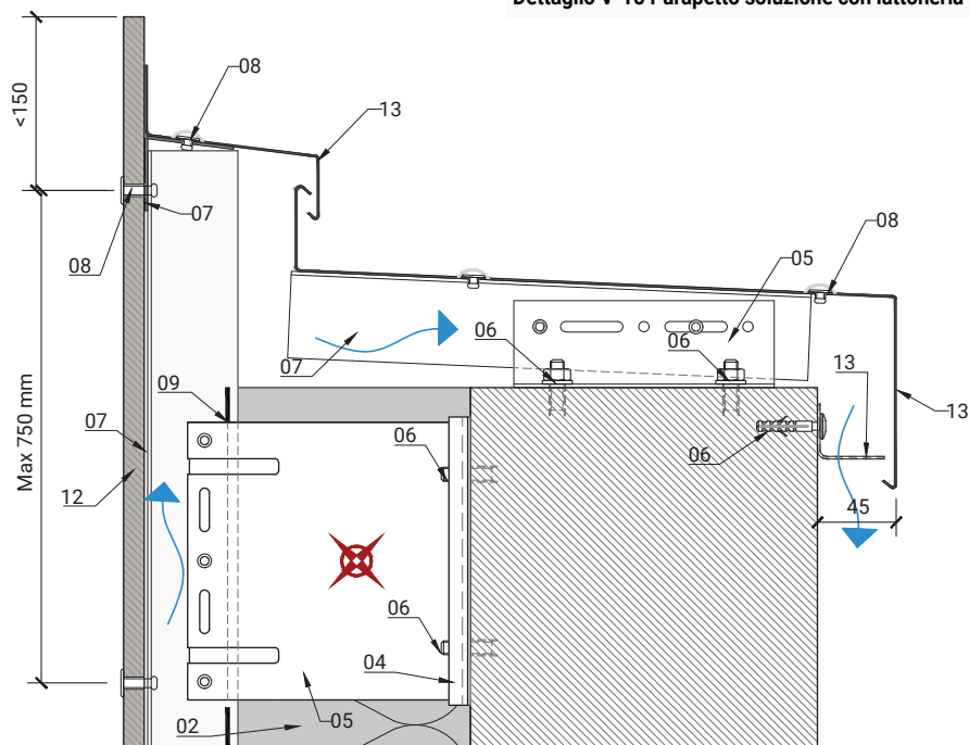
Dettaglio V-16 Parapetto con latteneria a vista
