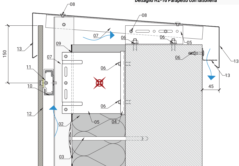
Dettaglio H2-16 Parapetto con lattoneria
