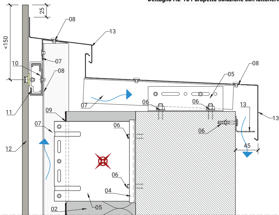
Dettaglio H2-16 Parapetto con lattoneria
