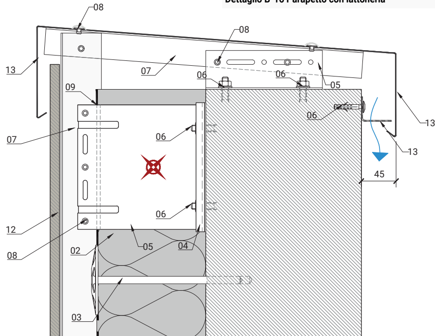
Dettaglio B-16 Parapetto con lattoneria
